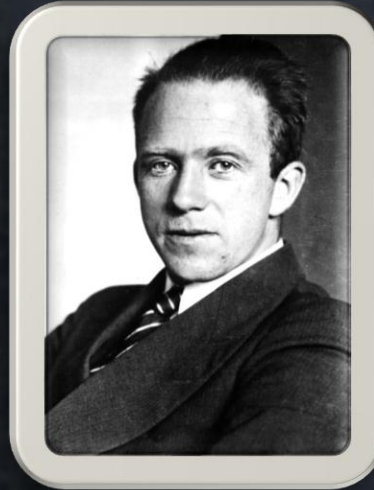
1932 Werner Heisenberg
